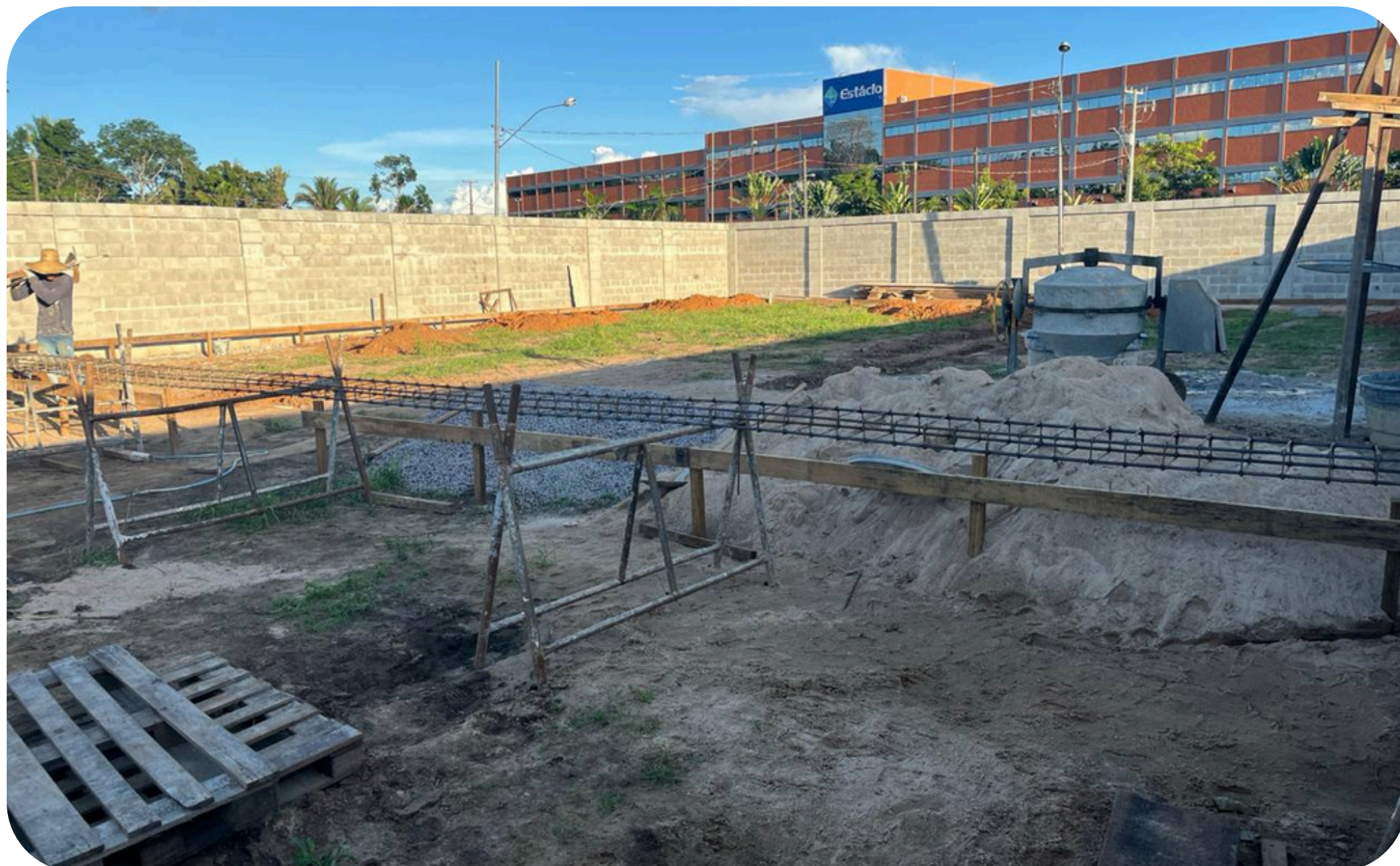
Imagem 01 - Armaduras vigas baldrames
