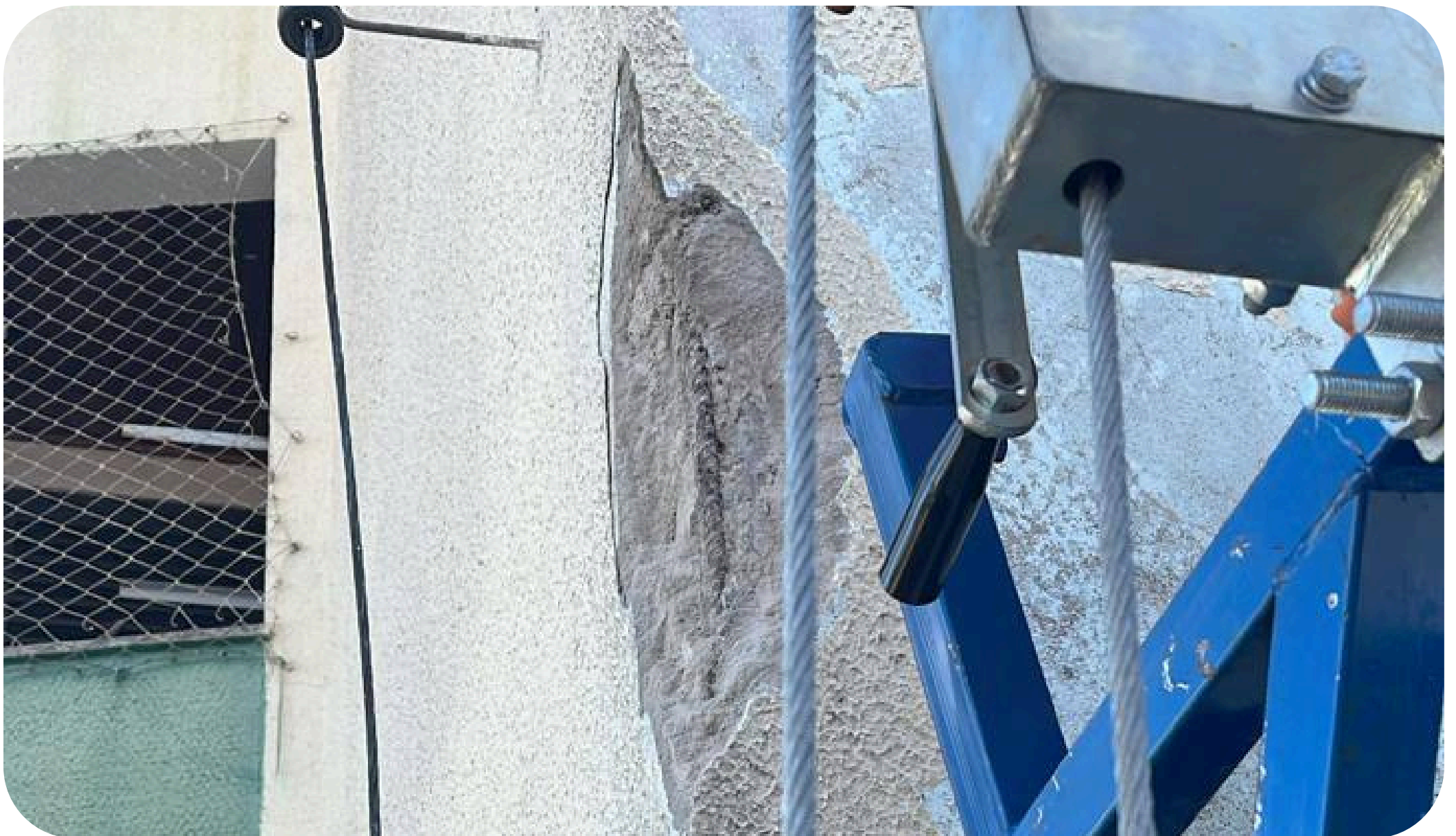
Imagem 03 - Pilar em destacamento de cobrimento
